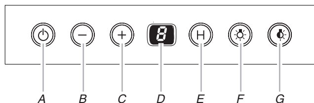
A. Fan motor on/off B. Decrease fan motor speed C. Increase fan motor speed D. Electronic display E. 10 minute timed boost F. Light G. Night light
