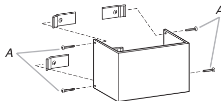
A. 4 vis à tête plate
