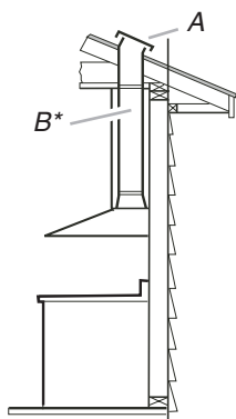
A. Bouche de décharge sur toit B. Conduit rond 6" (15,2 cm)*
