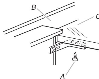
A. Lors de la fixation des brides sous le plan de travail, veiller à utiliser des vis de longueur appropriée, qui ne traverseront pas le plan de travail lors du serrage. B. Dosseret C. Plan de travail
