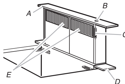
A. Garniture supérieure B. Bouton ON/OFF (marche/arrêt) C. Bouton de commande du ventilateur D. Embout E. Filtre ou filtres selon le modèle
