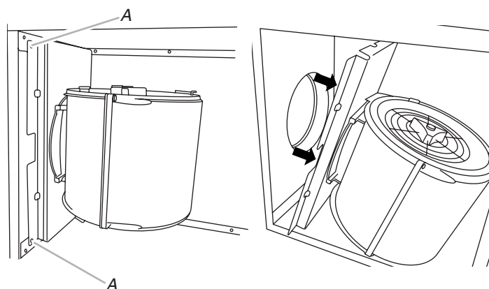
A. Vis de la bride de montage du moteur du ventilateur (2)
