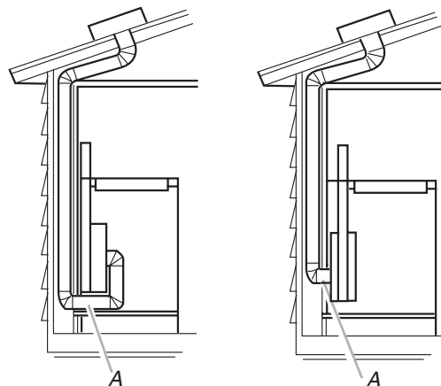
A. Conduit dia. 10" (25,4 cm)
