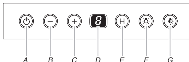
A. Bouton on/off (marche/arrêt) du ventilateur B. Diminuer la vitesse du moteur du ventilateur C. Augmenter la vitesse du moteur du ventilateur D. Affichage électronique E. Période d'accélération de 10 minutes F. Lampe G. Veilleuse
