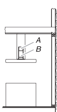
A. Raccord de déviation B. Conduit rond, dia. 6" (15,2 cm)
