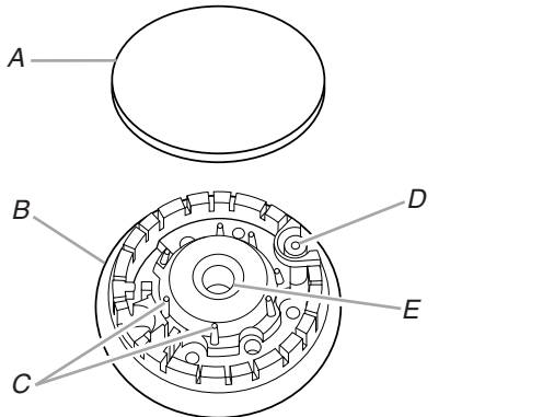
A. Tapa del quemador B. Base del quemador C. Espigas de alineación D. Encendedor E. Abertura del tubo de gas
