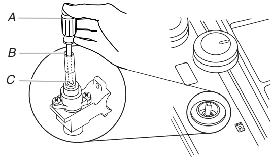
A. Tournevis à lame plate de 3/32" (n° 0 [2,0 mm]) (la longueur de la tige du tournevis doit être d'au moins 2" [5,1 cm]) B. Ouverture dans la tige du bouton de commande C. Emplacement de la vis de réglage
