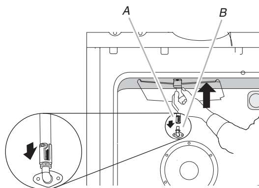
A. Gicleur de brûleur de gril B. Brûleur de cuisson au gril
