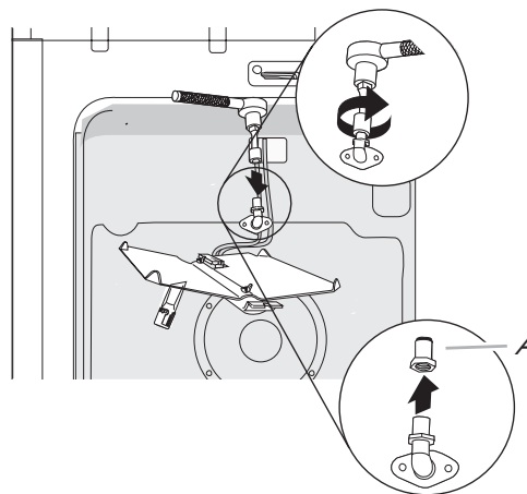
A. Injecteur femelle du brûleur de cuisson au grill pour gaz propane - numéro 0.037
