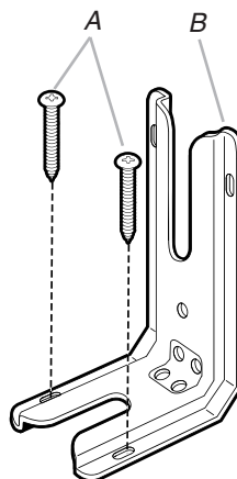
A. Vis n° 12 x \frac{15}{8} " B. Bride antibasculement
