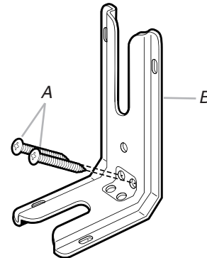
A. Vis n° 12 x \frac{15}{8} " B. Bride antibasculement
