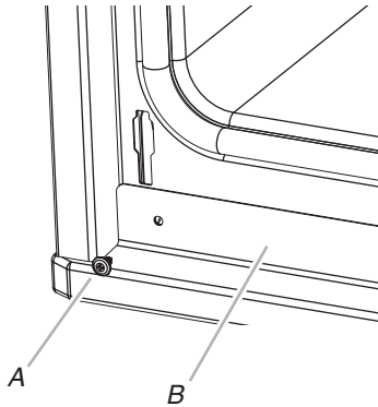
A. Vis n° 8-14 x \frac{3}{8} " B. Évén du four
