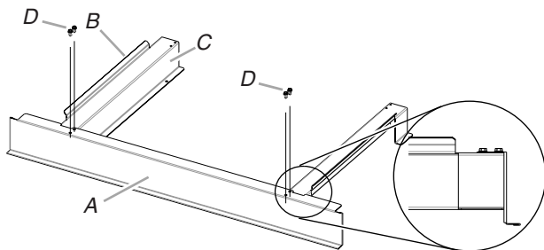
A. Évent inférieur B. Rebord de la barre de calage C. Barres de calage D. Vis rondelle à tête hexagonale de \frac{3}{8} "
