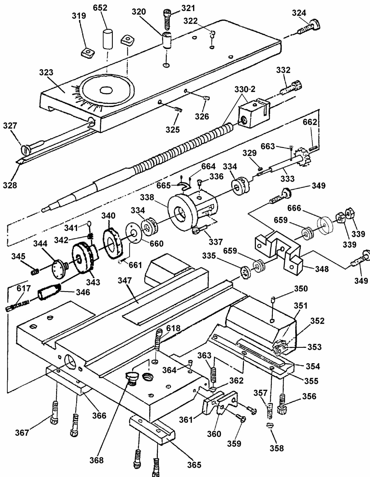
Saddle - Cross Slide Diagram / Diagramme du chariot longitudinal et transversal
