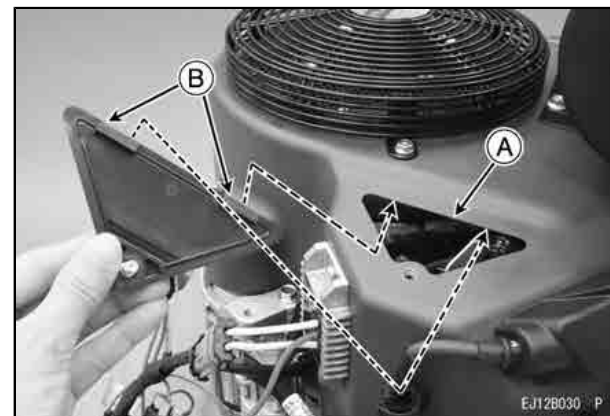
A. Inspection Port B. Tabs
