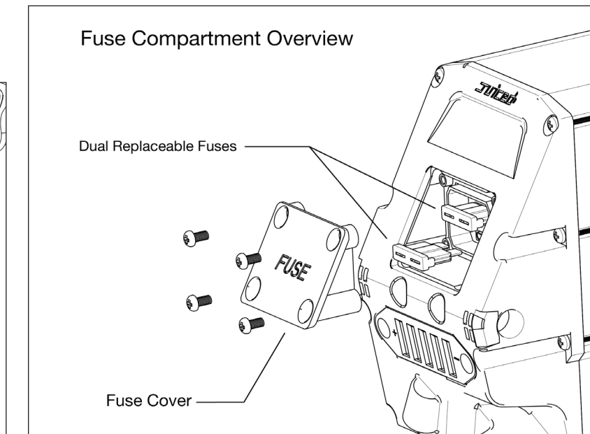
Fig. 8 - Fuse
