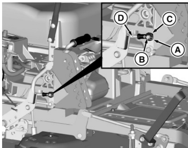
Maskinens högra sida visas med maskindelar borttagna för bättre vy. GXT002408—UN—30JUL15
