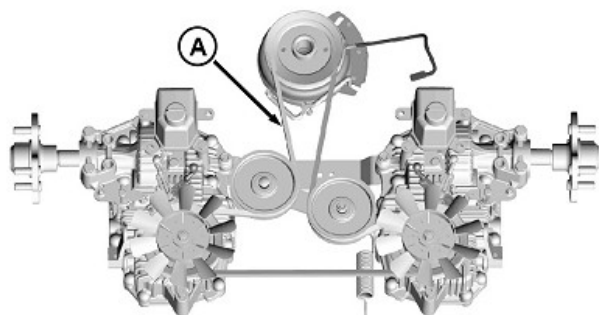
Komponenter sedda ovanifrån och framifrån. GXT002208—UN—09JUN15
