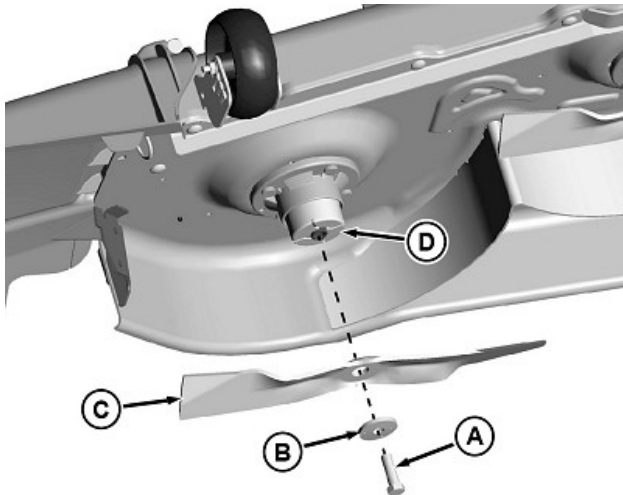
GXT002321—UN—18SEP15 48A klippdäck visas. 48HC-klippdäcket är liknande.
