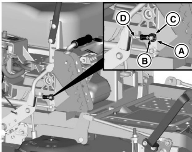
Lado direito da máquina mostrado com as peças da máquina retiradas para maior clareza da imagem. GXT002408—UN—30JUL15
