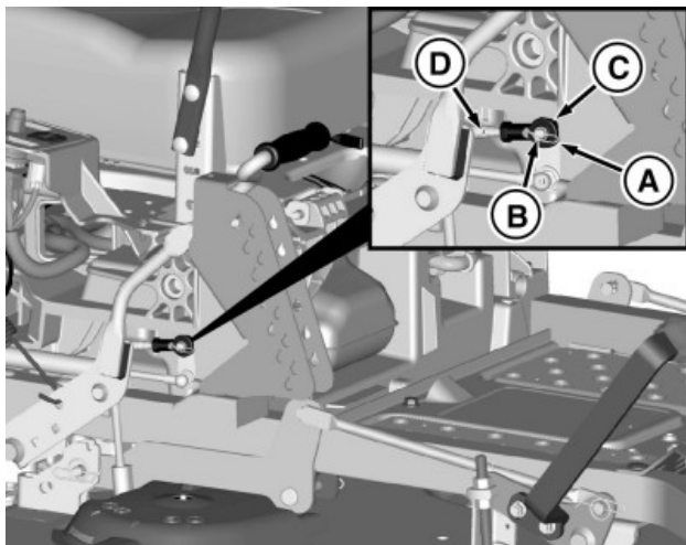
Z důvodu lepší názornosti je zobrazena pravá strana stroje s demontovanými díly.
