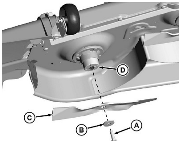
GXT002321—UN—18SEP15 Zobrazená je plošina 48A. Plošina 48HC je podobná.
