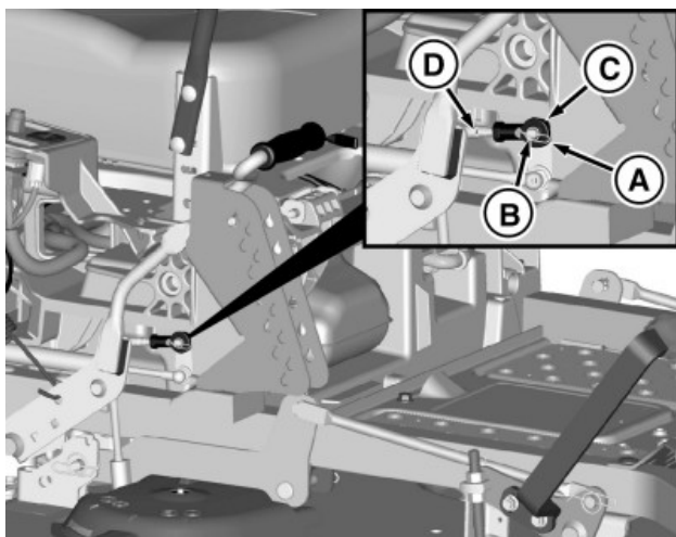
Pravá strana stroja je zobrazená s vybranými dielcami stroja kvôli lepšiemu prehľadu.
