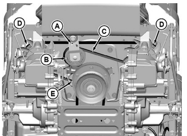
Vue du dessus des composants.
