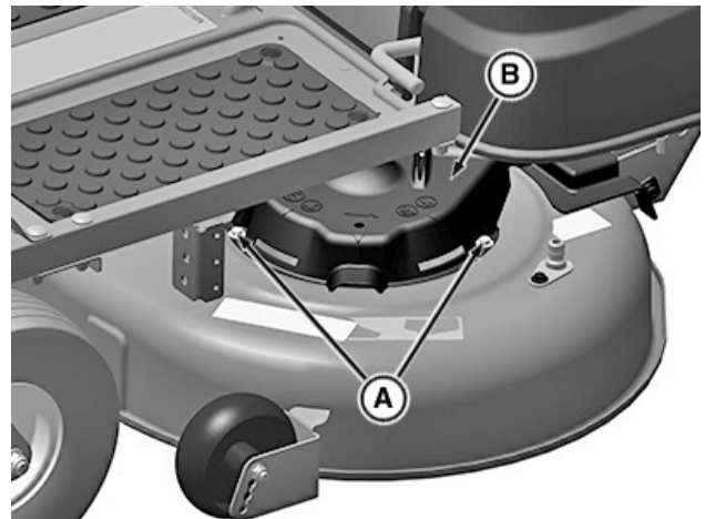
Avlägsna vänster spindelskydd
