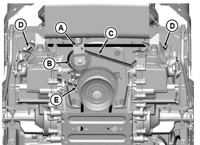
Componentes vistos desde abajo.
