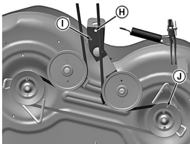
PY43380—UN—31MAY17 Plataforma exibida removida da máquina para uma melhor visualização.
