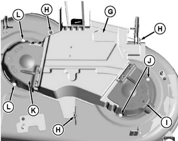
GXT002295—UN—17JUN15 Plataforma exibida removida da máquina para uma melhor visualização.
