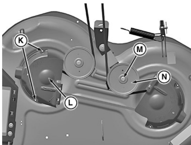
PY35592—UN—08JUN17 Plataforma exibida removida da máquina para uma melhor visualização.
