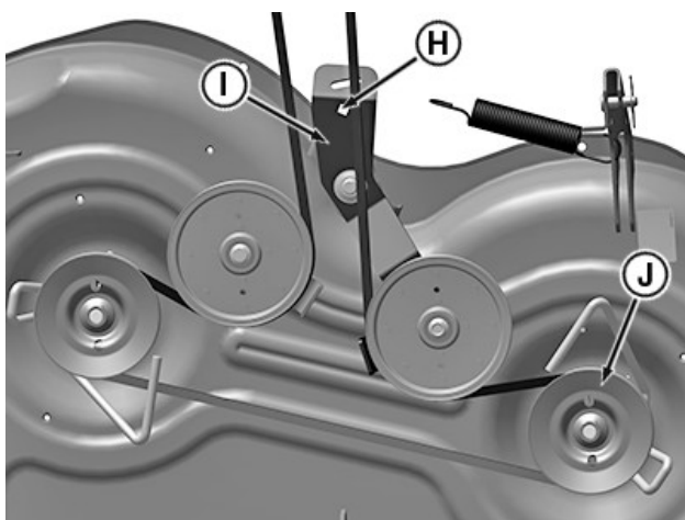
PY43380—UN—31MAY17 Plataforma exibida removida da máquina para uma melhor visualização.
