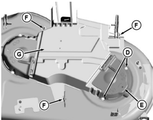
GXT002290—UN—17JUN15 Plataforma exibida removida da máquina para uma melhor visualização.
