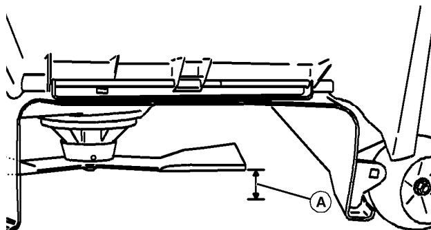
MXAL42867—UN—09APR13 Unité de coupe à éjection latérale illustrée
