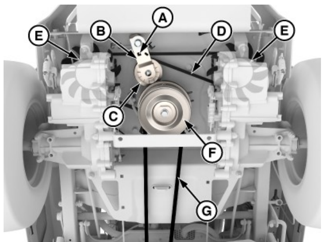
Componenti visti dal lato inferiore
