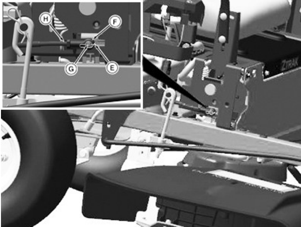
GX535583—UN—21APR22 Se muestra el lado derecho de la máquina con las piezas de la máquina extraídas para mayor claridad visual.
