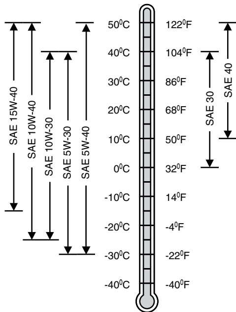
TS1744—UN—25AUG20 Viscosidades de aceite para rangos de temperatura del aire
