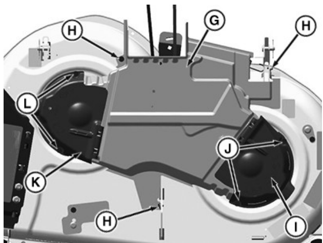
GX536016—UN—21APR22 Il piatto è stato rimosso dalla macchina a scopo illustrativo.
