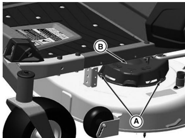
GXS35576—UN—21APR22 Rimozione copertura fusello del piatto tosaerba sinistro
