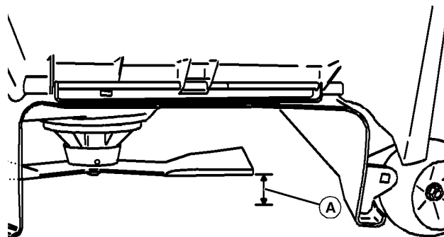
In figura: piatto tosaerba con scarico laterale
