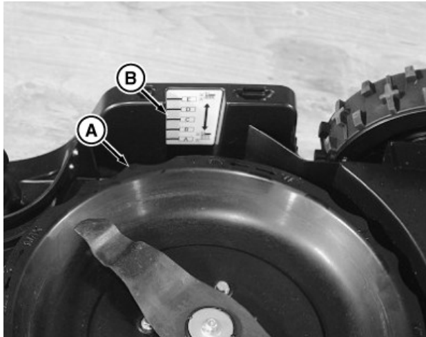
A—Protezione lama B—Etichetta altezza di taglio
