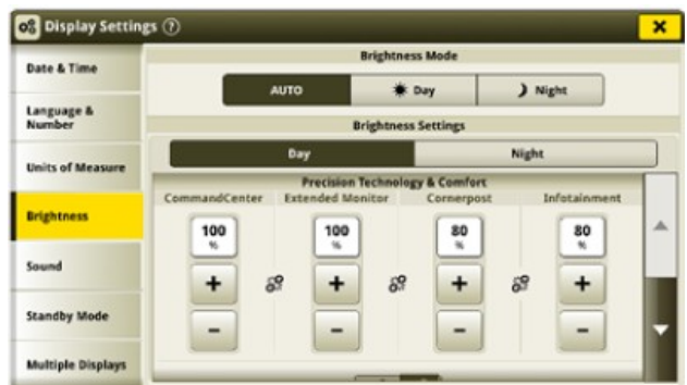
Pestaña "Brillo"
