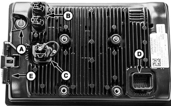
Componentes de la pantalla universal G5
