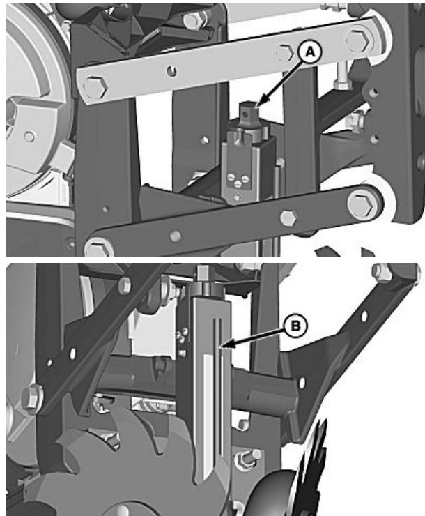
А—Поворотный регулятор
