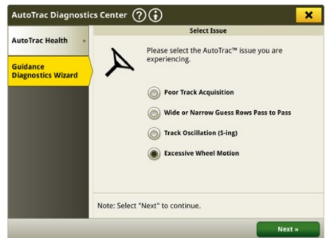
Pestaña de Asistente de diagnóstico de guiado
