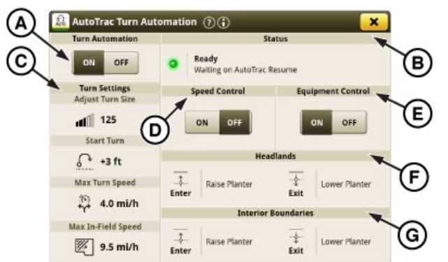
Страница с настройки на "Автоматизиране на завиването с AutoTrac на трактора"
