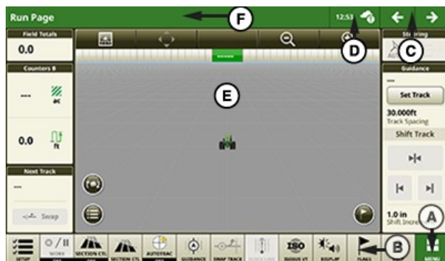
Pagina de rulare a afișajului
