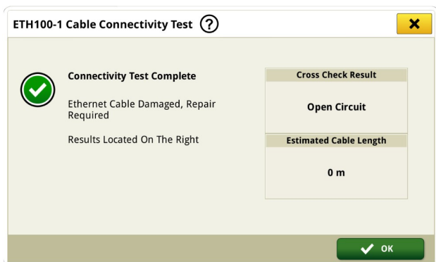
Перевірка підключення кабелю
