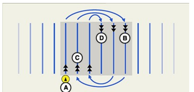
Giro de entrada en espiral con una superficie de 6
