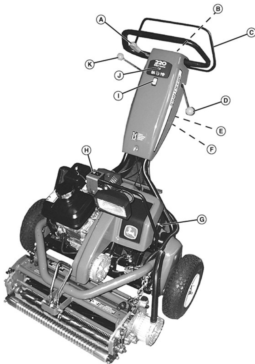
Органы управления
