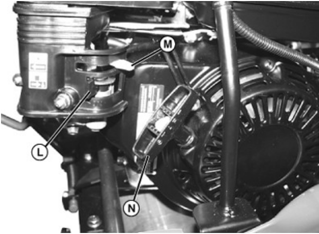
Comenzile motorului
