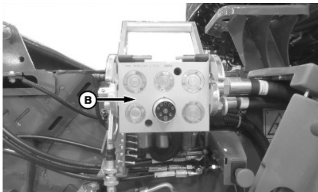
9-контактне з'єднання
