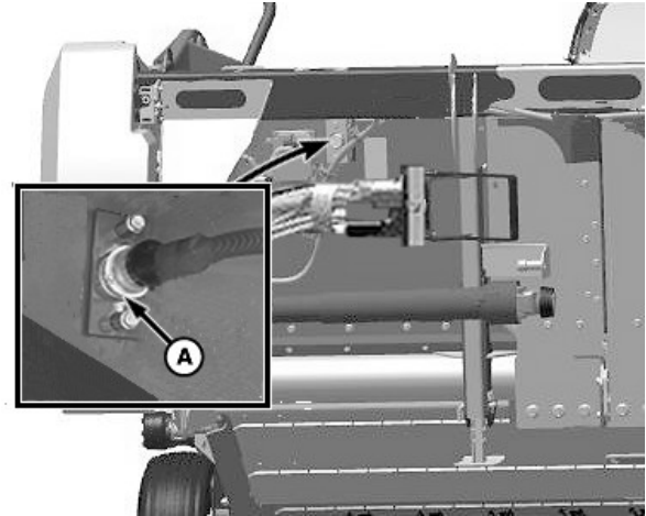
A—Elanslutningsfäste
