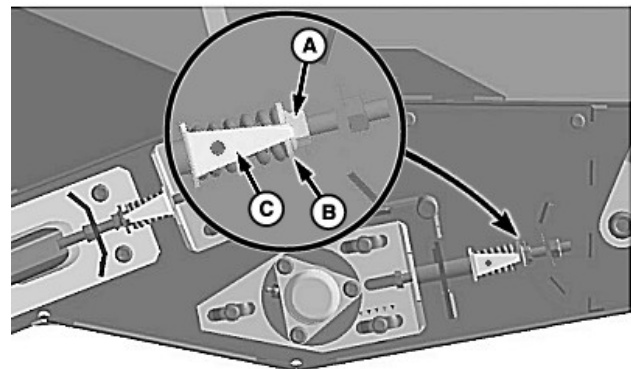
A—Регулировочная гайка B—Шайба C—Указатель
