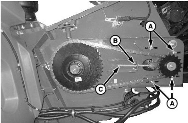
A—Гайка и крепежный болт (4 шт.) B—Стопорная гайка (2 шт.) C—Регулировочный болт
