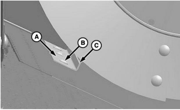
A—Монтажное отверстие с прорезями B—Болт C—Сталкиватель днища
