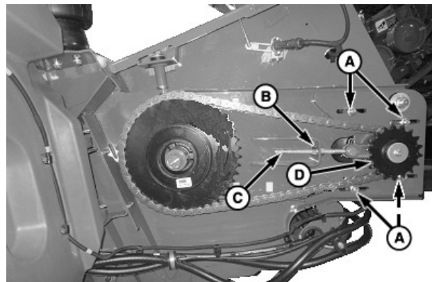
A—螺母和螺栓 (4 个) B—安全螺母 (2 个) C—调整螺栓 D—传动链轮
