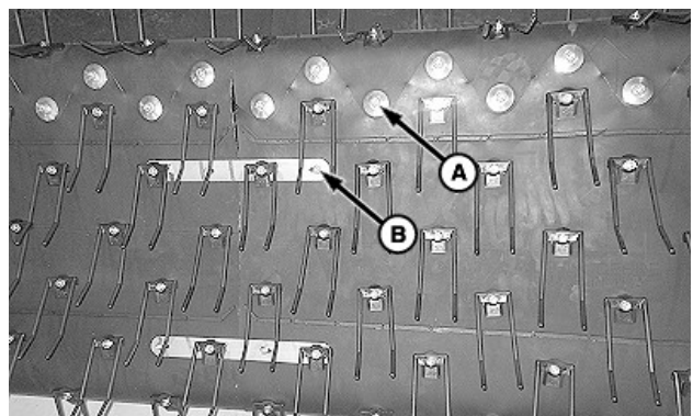
Передня стрічка
