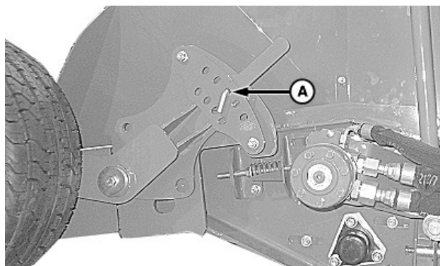
A—Центральне регулювання
