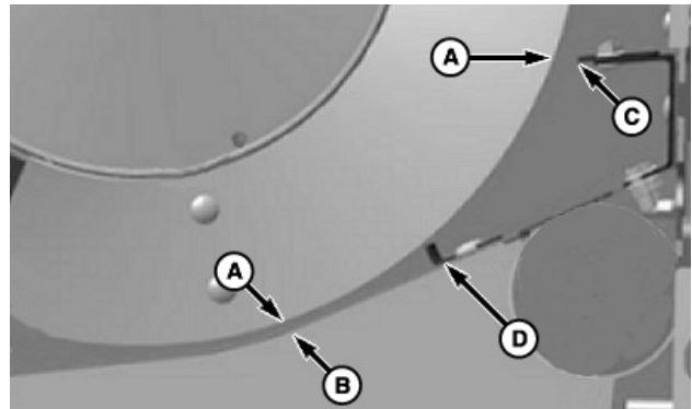
A—Espira B—Suelo (punto más cercano) C—Barra limpiadora trasera D—Barra limpiadora de suelo (referencia solamente)
