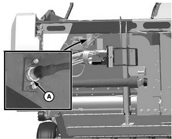
A—Soporte de conector eléctrico
