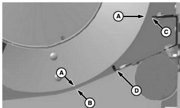
A—Spires de la vis d'alimentation B—Plancher (point le plus proche) C—Déflecteur du ramasseur arrière D—Déflecteur du ramasseur de la tôle de fond (pour référence seulement)
