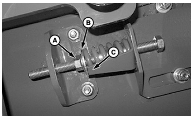
Courroie de ramasseur (courroie avant)
