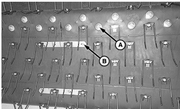
Courroie avant
