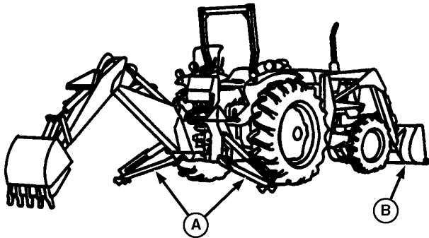
A—Stabilisateurs B—Benne de chargeur
