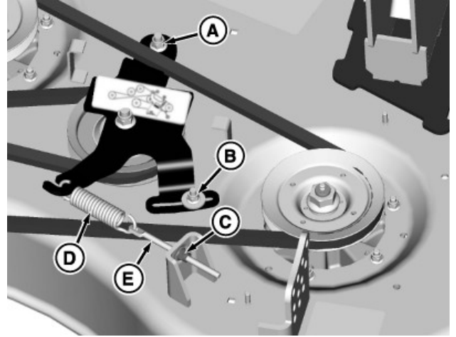
TCT008967—UN—27FEB14 사진: 60인치 측면 배출 데크 그림입니다.
