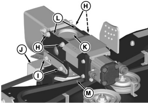
TCT008975—UN—27FEB14 사진: 60인치 GLC 측면 배출 데크 그림입니다.
