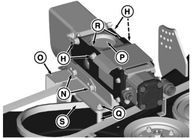
TCT009102—UN—27FEB14 사진: 72인치 GLC 측면 배출 데크 그림입니다.
