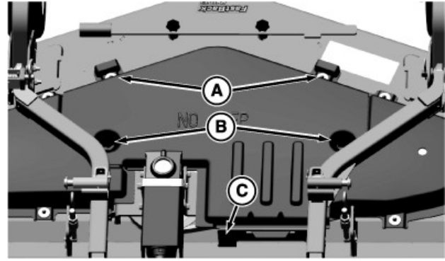
사진 참고: 72인치 후방 배출 모어 데크 그림.
