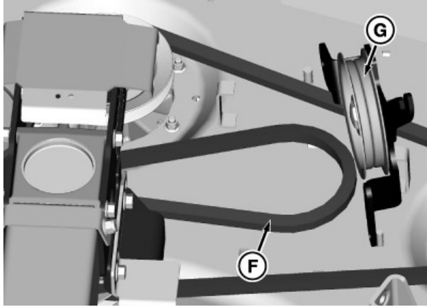
TCT008974—UN—07OCT13 사진: 60인치 GLC 측면 배출 데크 그림입니다.
