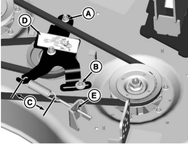
TCT008966—UN—27FEB14 60인치 측면 배출 데크 그림이며, 다른 데크도 이와 비슷합니다.
