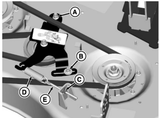
TCT008967—UN—27FEB14 사진: 60인치 GLC 측면 배출 데크 그림입니다.
