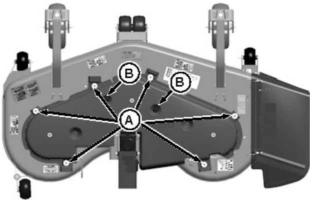
사진 참고: 60인치 측면 배출 모어 데크 그림.
