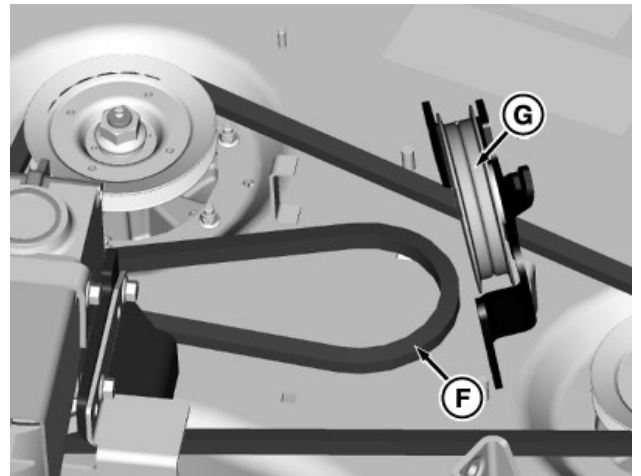
TCT008968—UN—07OCT13 사진: 60인치 측면 배출 데크 그림입니다.
