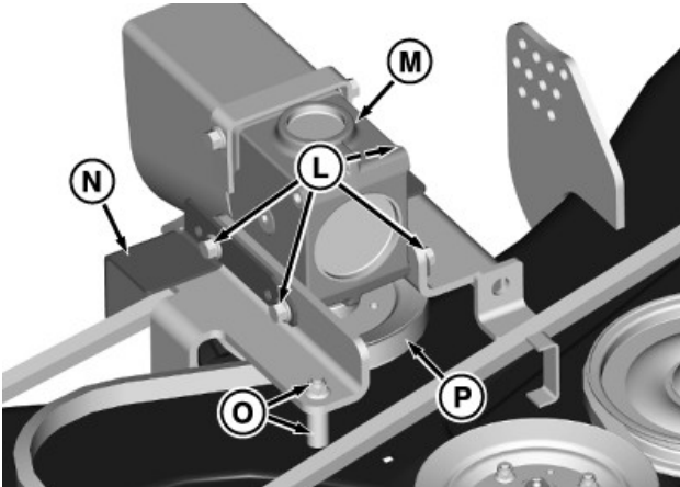
TCT008989—UN—27FEB14 사진: 72인치 측면 배출 데크 그림입니다.
