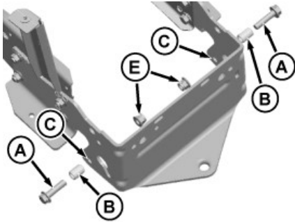
Az ábra az X394 és az X500 modellt mutatja. GXT002225—UN—14JUL15
