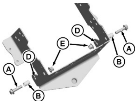
Az ábrán az X300 modell látható.
