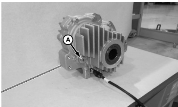
A88356—UN—03NOV15 Aceite de la caja de engranajes
