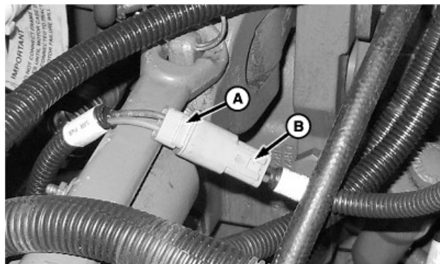
A83273—UN—12AUG14 Conexión del apero al tractor
