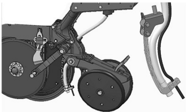
Aplicador en surco
