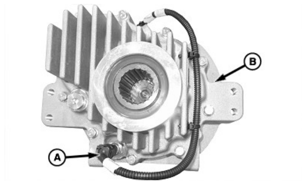
A—Grupo de cables de temperatura B—Caja de engranajes
