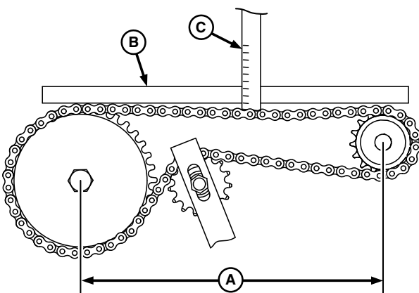
A70496—UN—31JAN11 Cadena de transmisión con polea tensora
