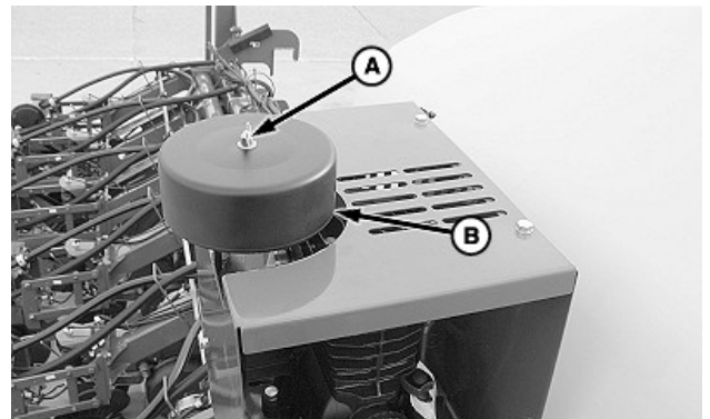
Filtro de aire montado en el compresor (compresor hidráulico)
