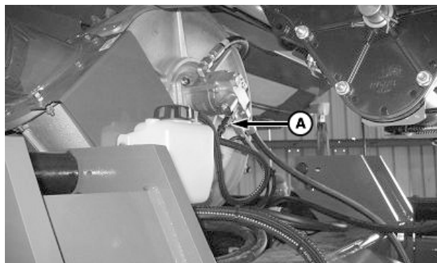
A74976—UN—23MAR12 A—Grupo de cables del solenoide del CCS™
