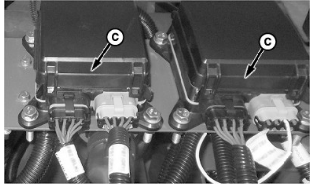
Cajas de fusibles dobles
