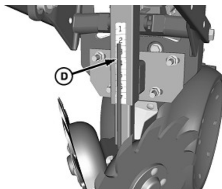
Limpiador de hileras montado en la unidad
