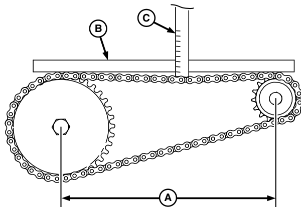
A70495—UN—31JAN11 Cadena de transmisión sin polea tensora
