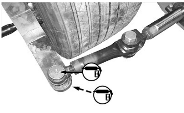
Мост заднего рулевого управления
