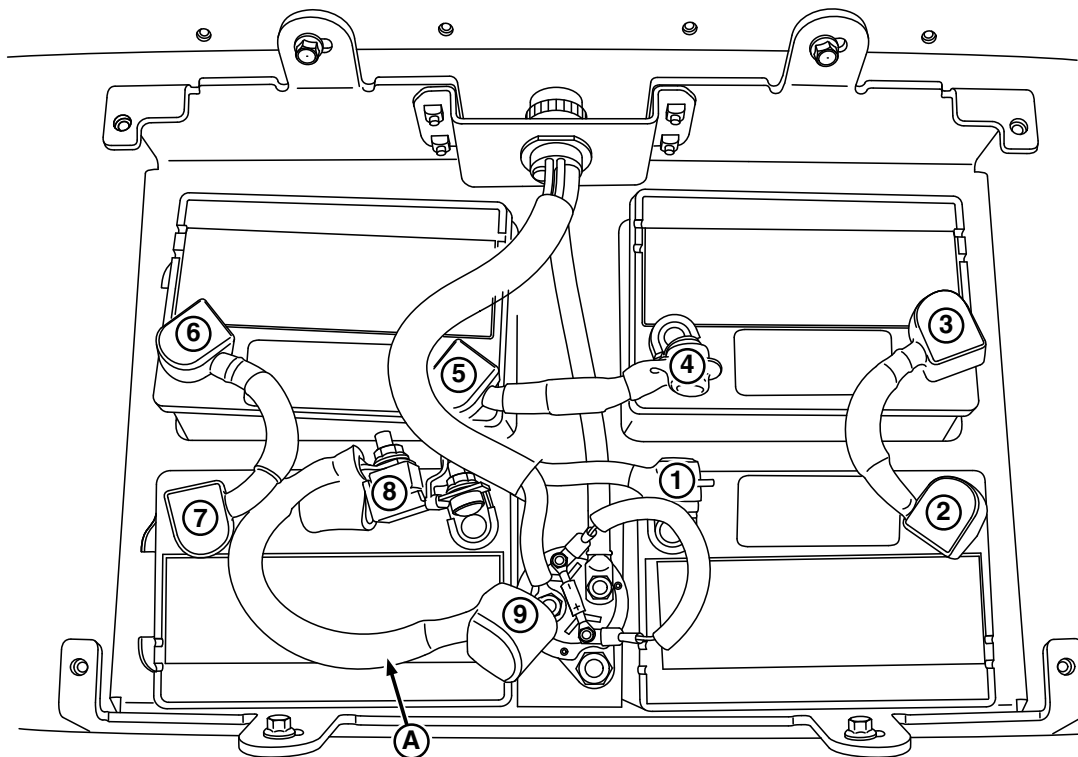
Последовательность установки
