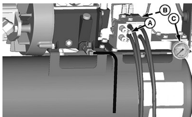
Гидравлический компрессор
