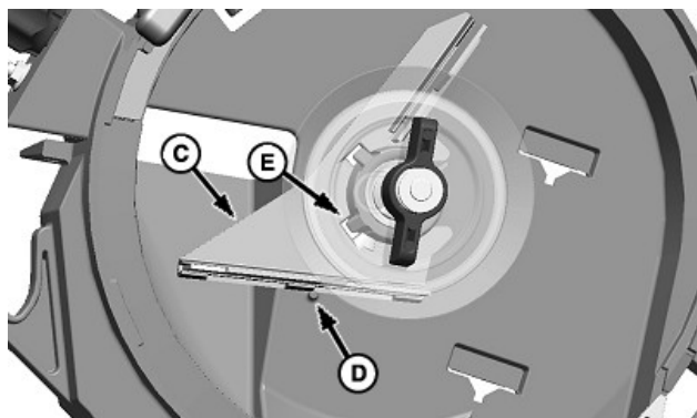
Задняя щетка
