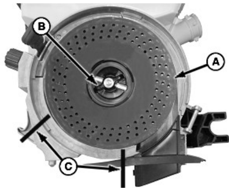
А—Высевающий диск В—Ступица С—Сектор контроля
