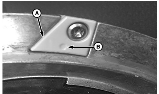
Керамическая износная накладка дозатора
