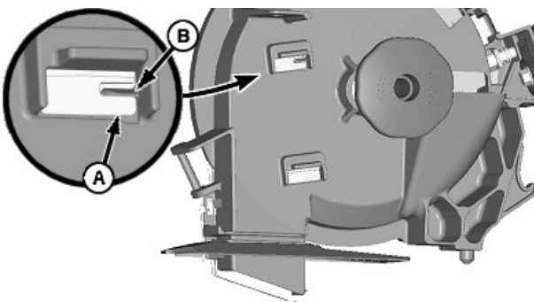
А77792—UN—01MAY13 Задняя часть дозатора для семян
