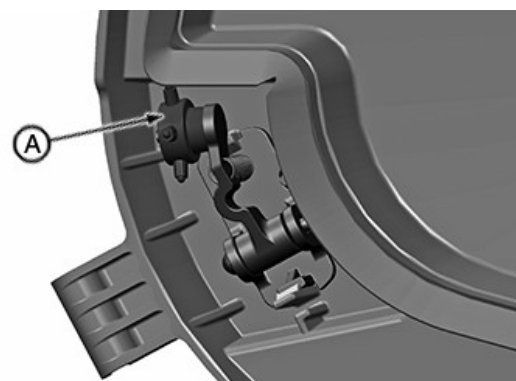
А—Колесо выталкивателя семян
