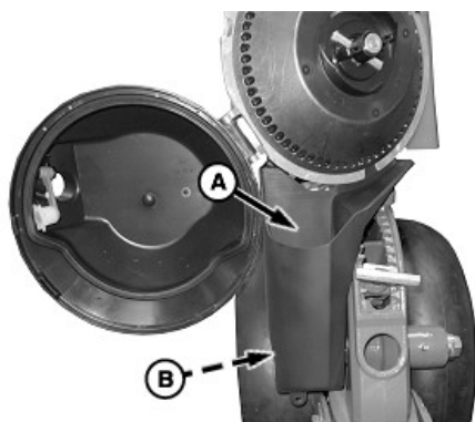
A—Очистной поддон B—Рычаг копирующего колеса
