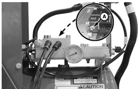
Ручная блокировка выхлопа
