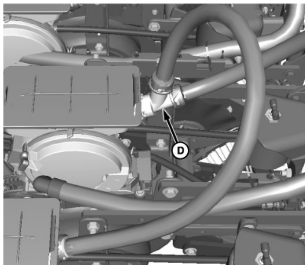
Соединительный шланг
