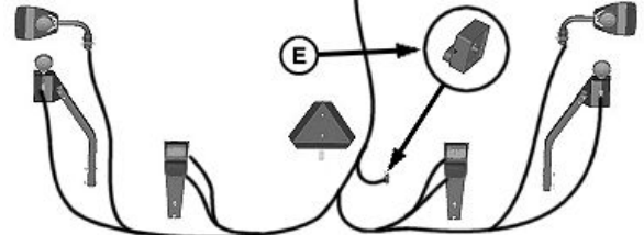
Configuración de luces en sembradoras integrales
