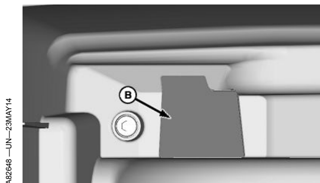
Posición cerrada
