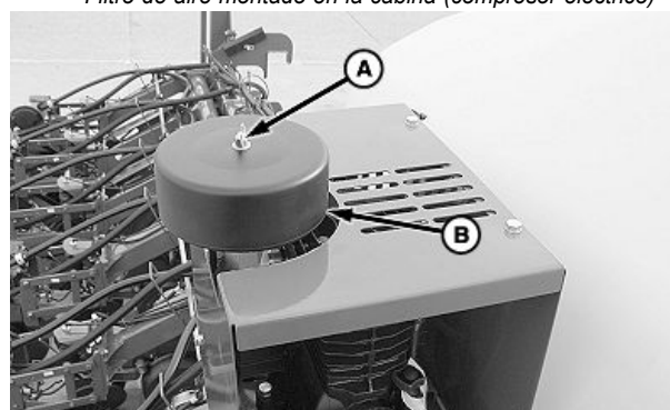
Filtro de aire montado en el compresor (compresor hidráulico)
