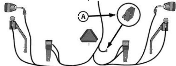
Configuración de luces—Estilo A
