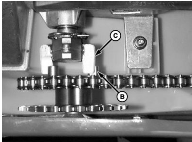
Mandos desalineados
