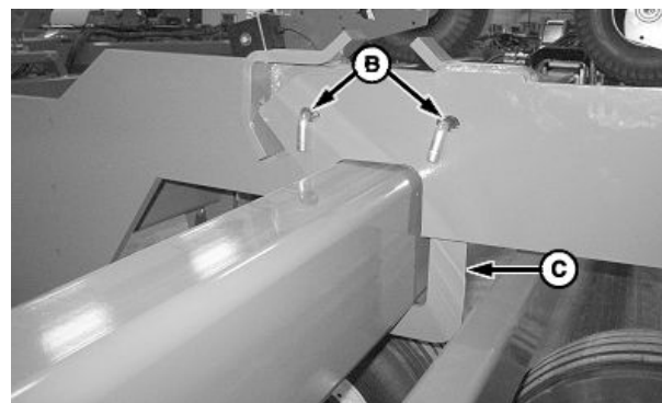
A—Pasador tipo beta (se usan 2) B—Pasador (se usan 2) C—Collar
