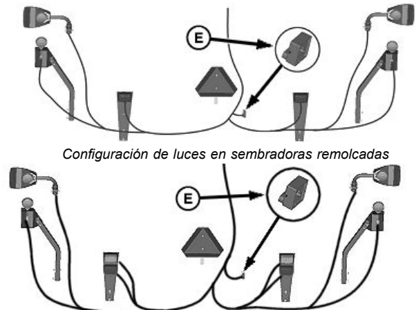
Configuración de luces en sembradoras integrales
