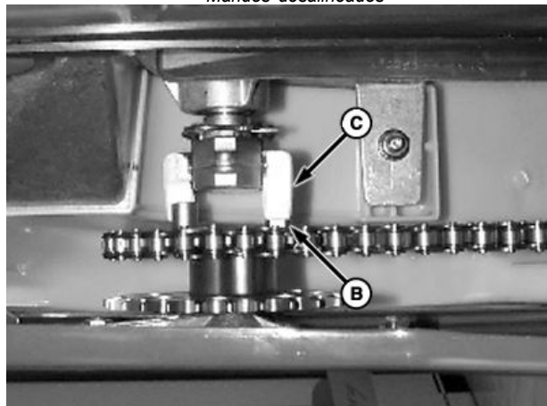
Mandos alineados
