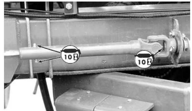
Ejes sembradores
