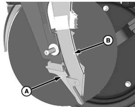
A —Dispozitiv de protecție tub B —Tub de însămânțare de însămânțare
